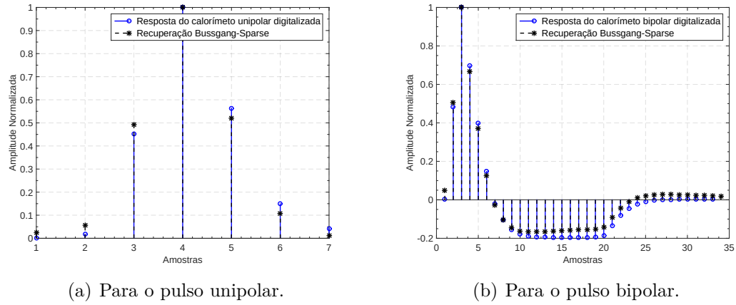
Figura 52 – Recuperação do pulso característico para o cenário sem ruído.
