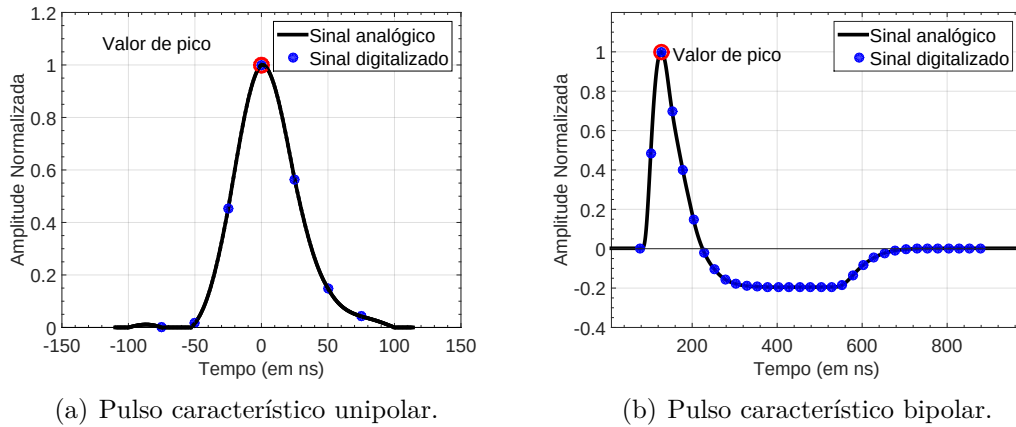
Figura 30 – Respostas ao impulso consideradas na Toy Monte Carlo Simulation .
