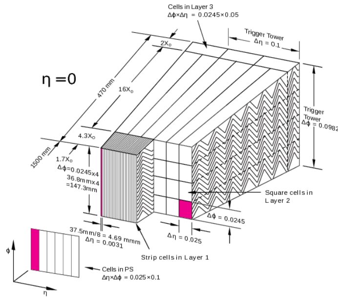
Figura 6 – Granularidade do LAr.
