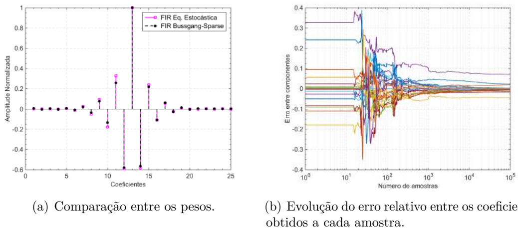
Figura 64 – Cenário de ocupância em 30 % com inserção de ruído.
