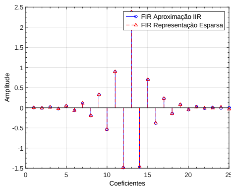
(a) Para o pulso unipolar.
