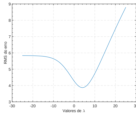
Figura 40 – Variação do RMS do erro para cada \lambda para uma ocupância de 30%.
