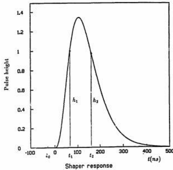
Figura 20 – Amostras do pulso de referencia do calorímetro eletromagnético do ZEUS no experimento HERA.
