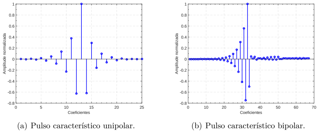
Figura 35 – Coeficientes do filtro FIR de deconvolução projetado por meio da aproximação ao sistema inverso para cada tipo pulso.
