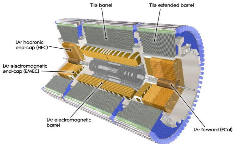
Figura 5 – O sistema de calorimetria do ATLAS.
