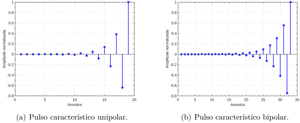
Figura 34 – Respostas ao impulso de g'_{01}[n] atrasadas para tornar o sistema causal.
