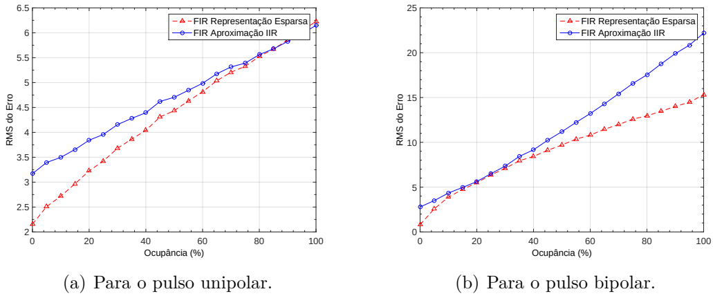
Figura 43 – Comparação entre a representação esparsa e a técnica de aproximação do sistema inverso em função da ocupância e relação sinal ruído em aproximadamente 28 dB.
