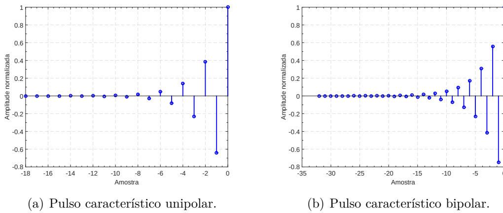
Figura 32 – Respostas ao impulso de g'_{01}[n] após a inversão de sua região de convergência.
