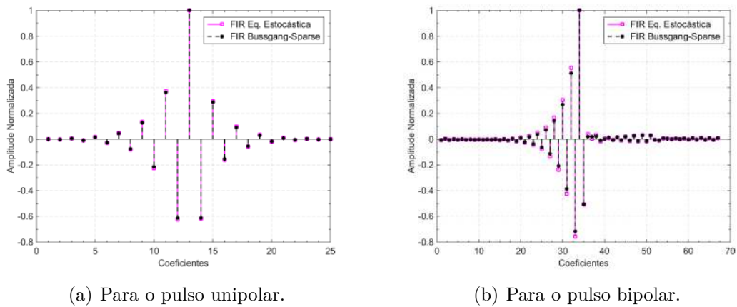
Figura 48 – Comparação entre os coeficientes finais obtidos pelo método Busgang-Sparse e o de Equalização estocástica para um cenário de ocupância em 1% sem ruído.
