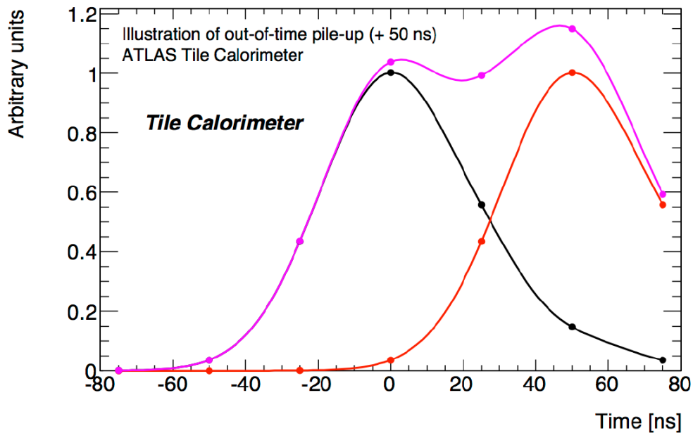
Figura 16 – O efeito de empilhamento de sinais.
