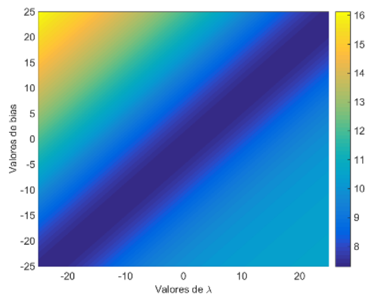
Figura 45 – Variação do RMS do erro em função do bias e valores de \lambda .
