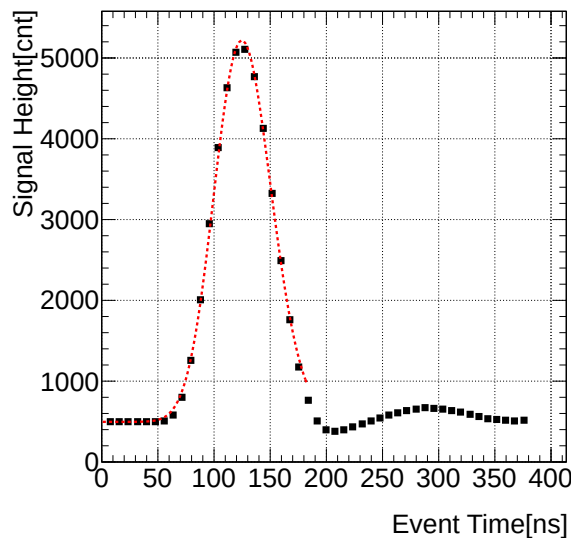
Figura 19 – Amostras do pulso de referencia do calorímetro eletromagnético CsI no experimento KOTO.
