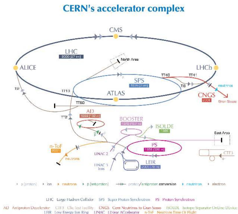
Figura 1 – O complexo de aceleradores do CERN.
