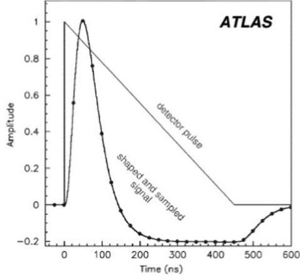
Figura 7 – Pulso característico do LAr e seu pulso de referência.
