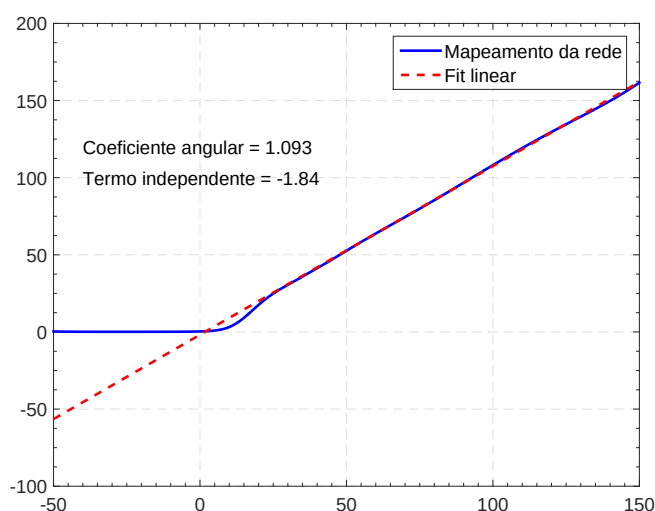
Figura 28 – Mapeamento da função por meio da rede estimadora e fit linear.
