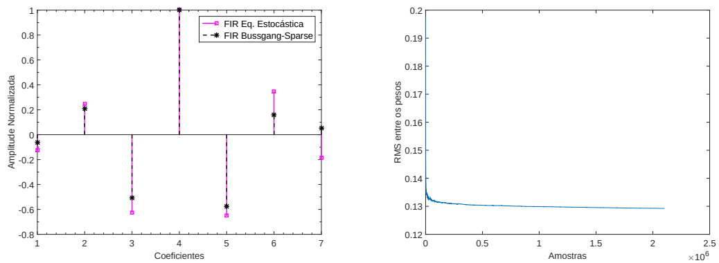
Figura 59 – Análise para célula E4 com \mu = 90 .
