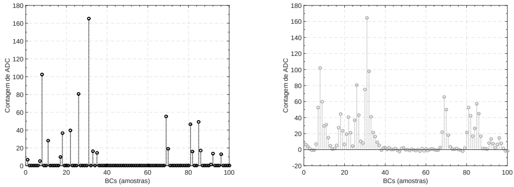
(c) Sorteio de amplitudes de energia depositadas (d) Sinal simulado da saída do calorímetro unipolar.
