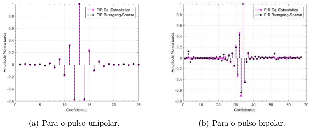
Figura 50 – Comparação entre os coeficientes obtidos pelo método Busgang-Sparse e o de Equalização estocástica para um cenário de ocupância em 30% e com ruído.
