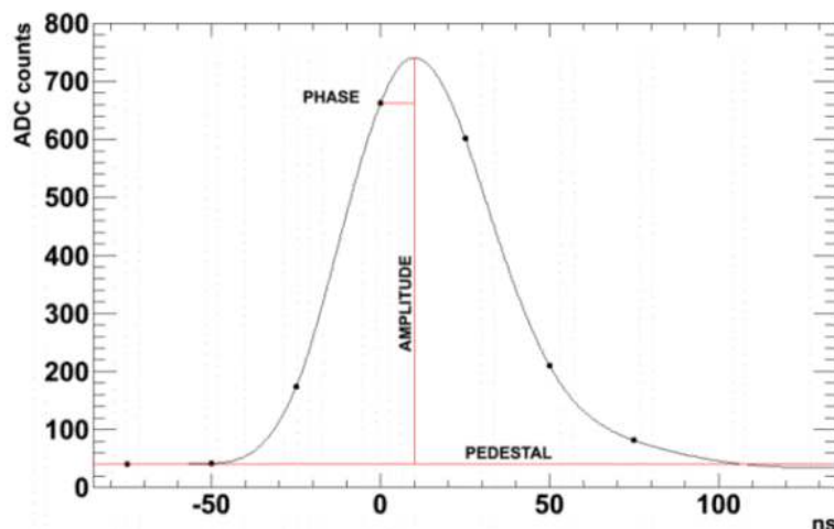
Figura 9 – Pulso característico do TileCal.
