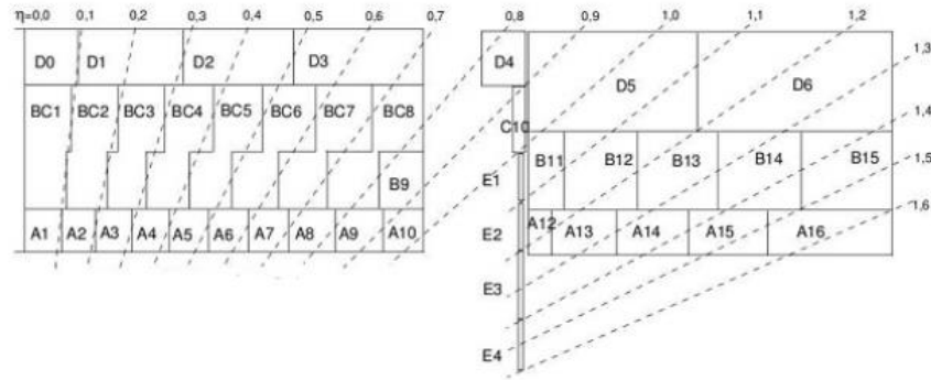
Figura 8 – Segmentação do TileCal.
