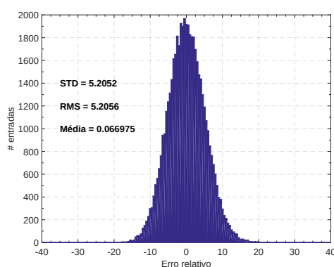
Figura 38 – Distribuição do erro de estimação para o pulso bipolar após a correção do bias .
