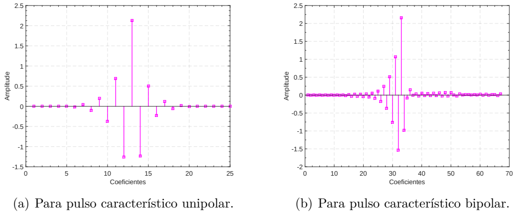
Figura 36 – Coeficientes do filtro FIR de deconvolução projetados a partir da técnica de equalização estocástica.
