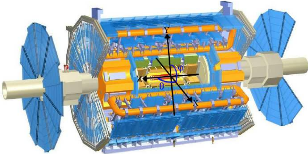
Figura 4 – O sistema de coordenadas do ATLAS.
