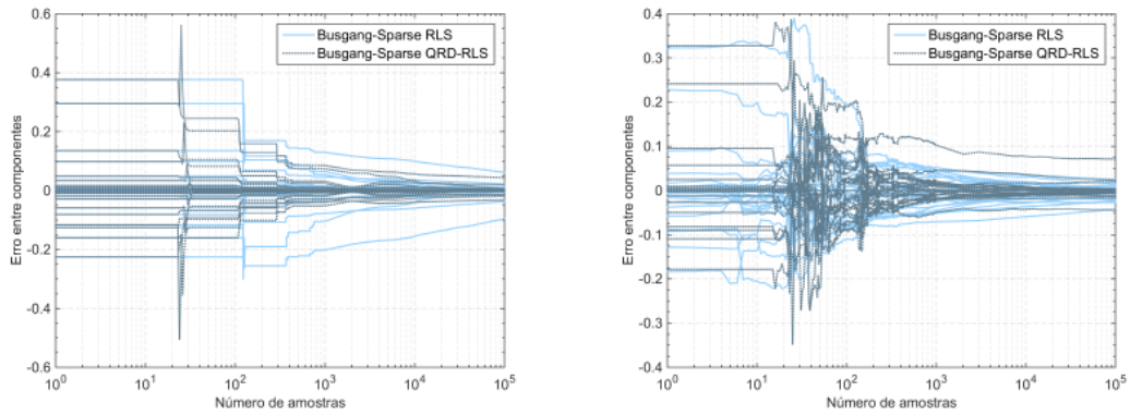
(a) Cenário de ocupância em 1 % sem inserção de ruído. (b) Cenário de ocupância em 30 % com inserção de ruído.
