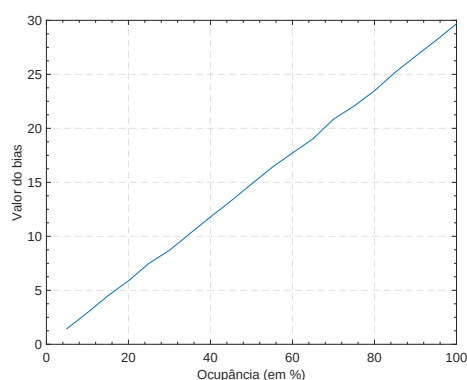
Figura 39 – Variação dos valores do bias em função da ocupância para o pulso bipolar.
