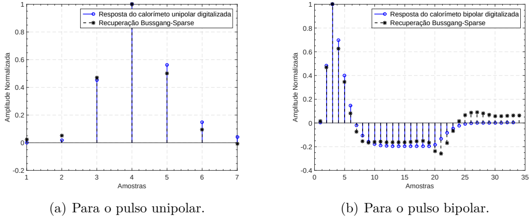
Figura 53 – Recuperação do pulso característico para o cenário de ocupância fixada em 30% e adição de ruído.
