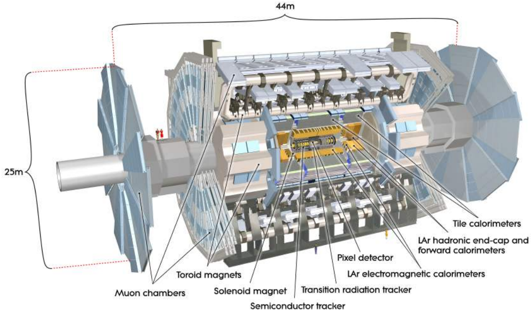
Figura 3 – O ATLAS e seus componentes.
