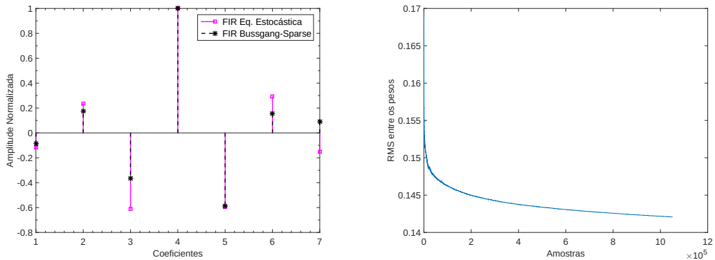
Figura 57 – Análise para célula E4 com \mu = 50 .
