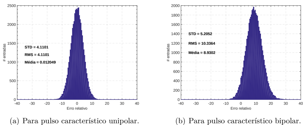
Figura 37 – Distribuição do erro de estimação para cada tipo de pulso, utilizando os pesos projetados que são mostrados na Figura 36.
