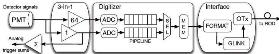
Figura 13 – Arquitetura do TileCal durante as Run I e Run II.
