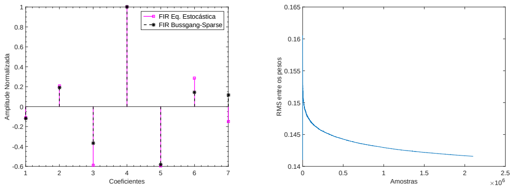
(a) Comparação entre os pesos do filtro por equa- (b) Evolução do erro RMS entre os pesos em lização estocástica e do algoritmo cego Bussgang- função do número de amostras. Sparse.
