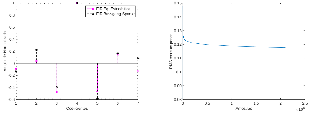
Figura 58 – Análise para célula A2 com \mu = 90 .
