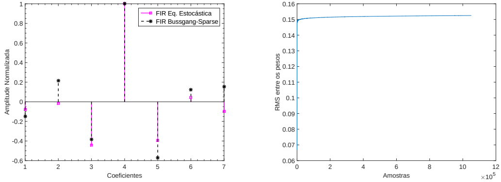
Figura 56 – Análise para célula A2 com \mu = 50 .
