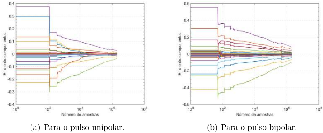
Figura 49 – Evolução do erro relativo entre os coeficientes obtidos a cada amostra para o cenário de ocupância em 1% sem ruído.
