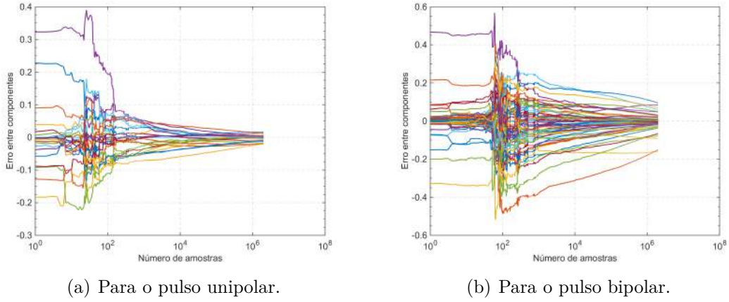
Figura 51 – Evolução do erro relativo entre os coeficientes obtidos a cada amostra para o cenário de ocupância em 30% e com ruído.
