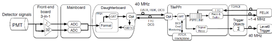
Figura 14 – Arquitetura do TileCal para a Fase II de atualização.
