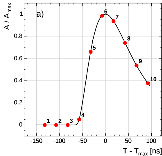
Figura 18 – Amostras de referencia do calorímetro eletromagnético do CMS.
