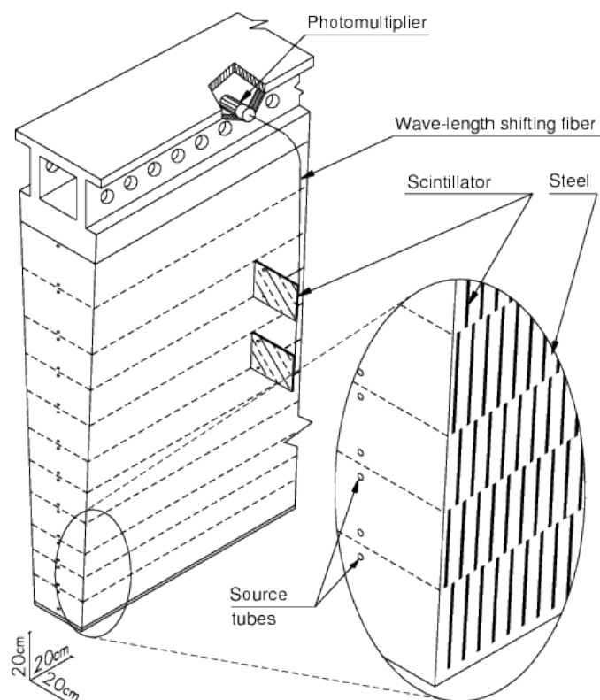
Figura 10 – Módulo do TileCal.
