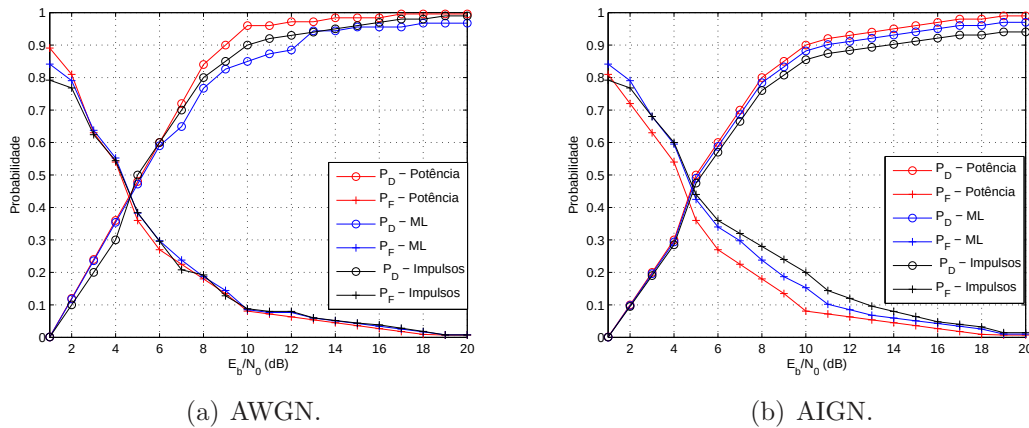
Figura 15: Curvas P_D e P_F \times E_b/N_0 para o canal PLC indoor 1.
