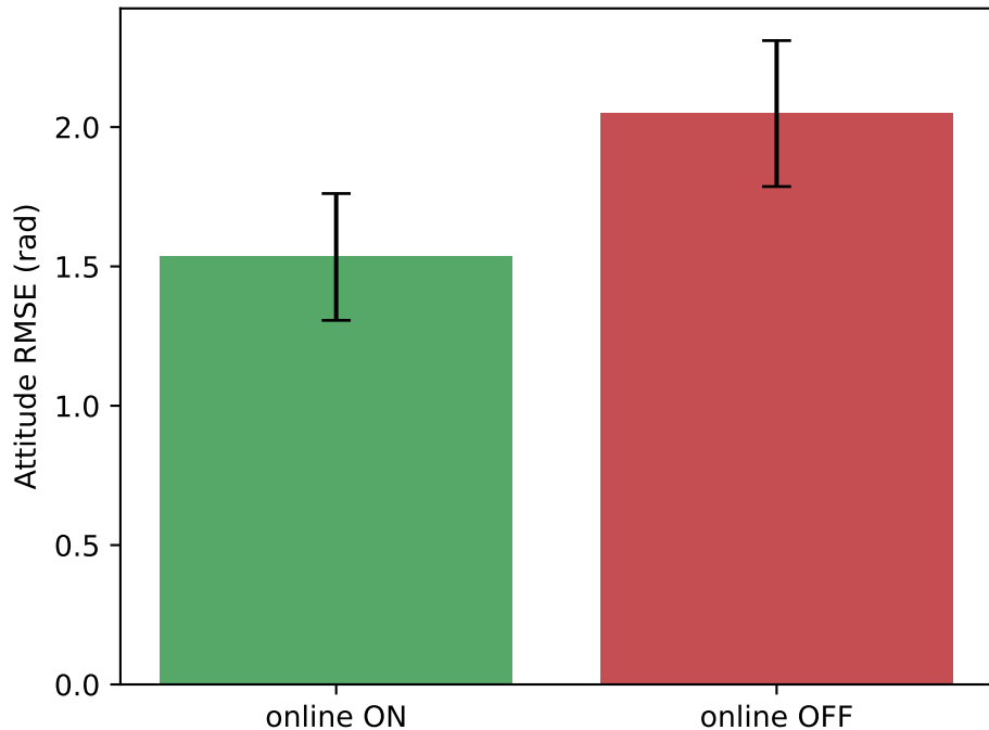
Ablation: RTRL-RTU Online Updates (Fault Scenario)
