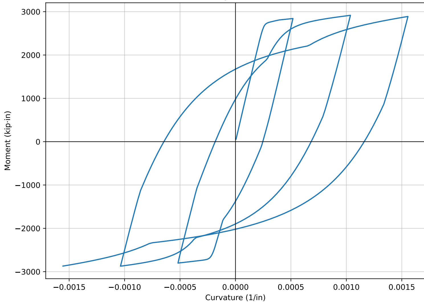
Moment-Curvature Diagram (Steel 02-Concrete 01)
