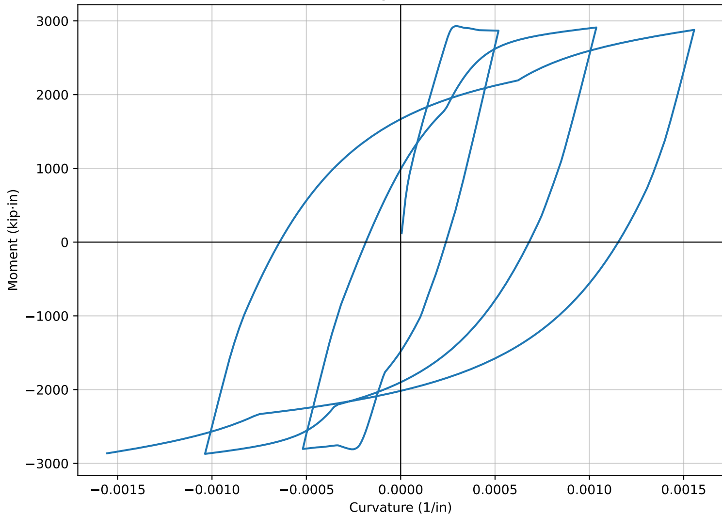
Moment-Curvature Diagram (Steel 02-Concrete 02)
