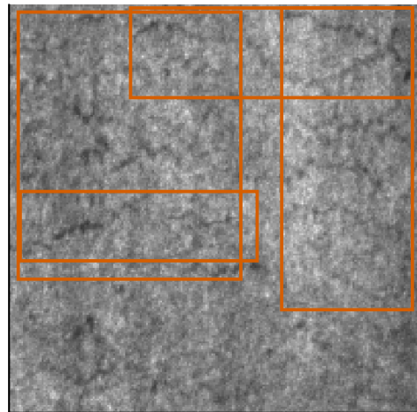
00 input
