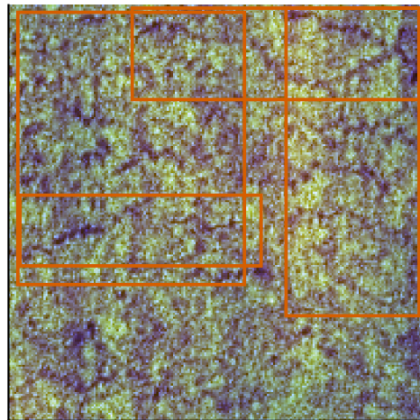
04 cce composite
