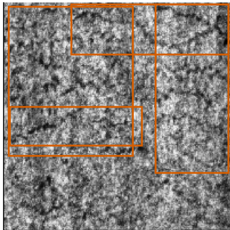
02 ch1 clahe
