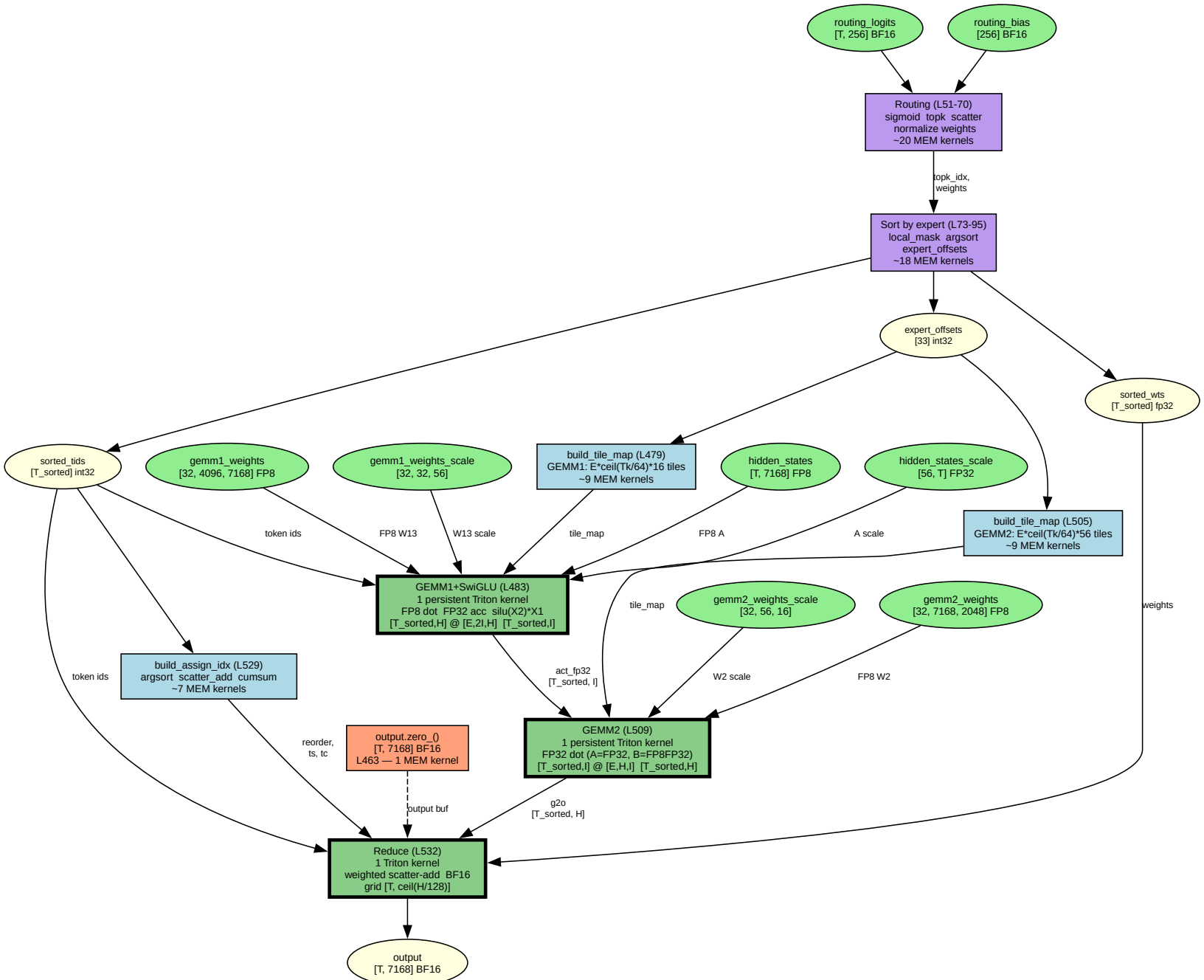
kernel.py (Triton) — Critical Path DAG
