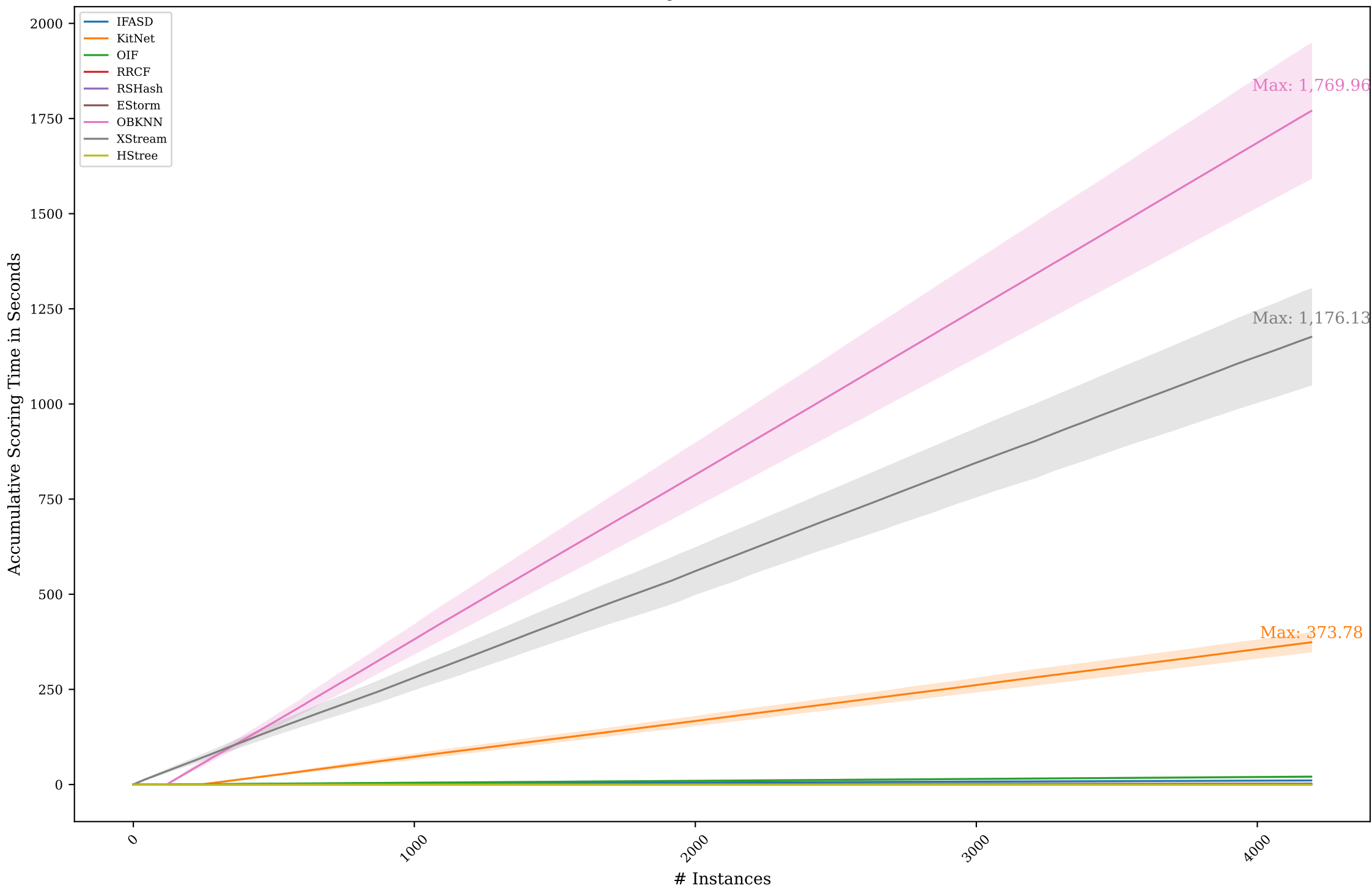
Scoring Time: Scenario A5
