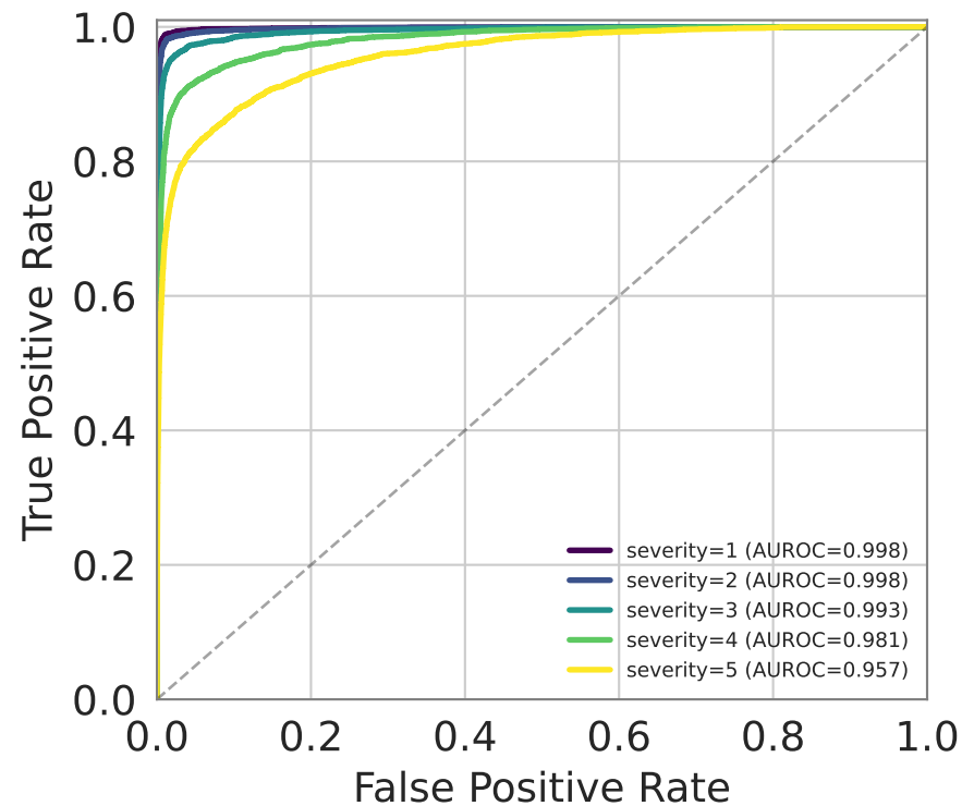
SNGP
