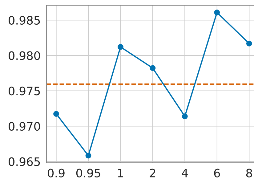
Precision (macro)
