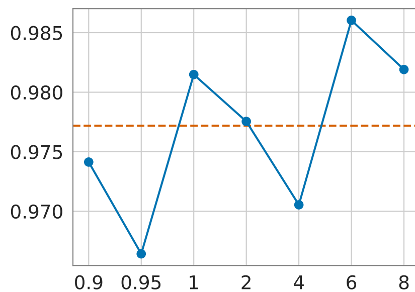
F1 (macro)
