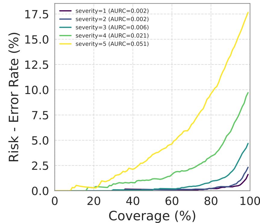
SNGP
