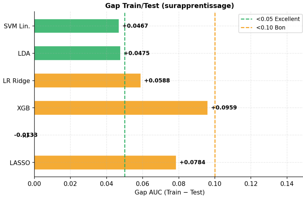
Figure 5.4 — Train-test AUC gap per model — vert < 0.05 (excellent), orange < 0.10 (acceptable). SVM Linéaire : gap le plus faible (0.047).
