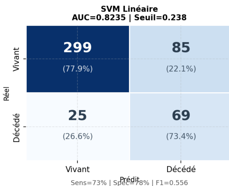
Figure 5.8 — Confusion matrix — SVM Linéaire (AUC = 0.8235, seuil = 0.238).
