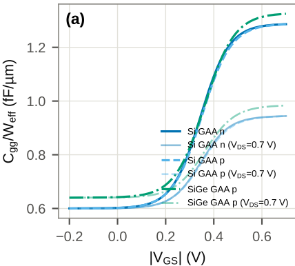
Si / SiGe nanosheets
