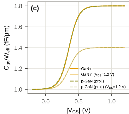
GaN
