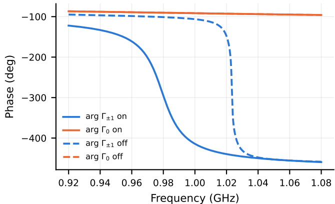
(b) Eigenmode reflection phase
