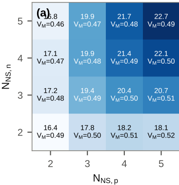
CFET-Si: f_{RO} (GHz)
