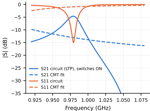
(a) Unmodulated: CMT parameter extraction
