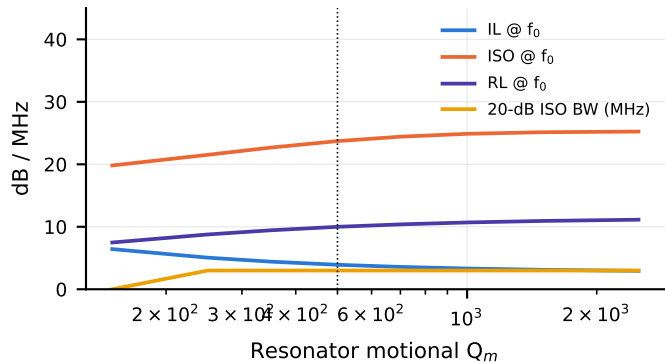
(d) Resonator quality factor
