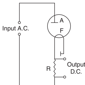
Fig. 22.26 Rectifier.
