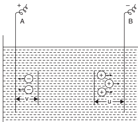
Fig. 9.4 Voltameter.
