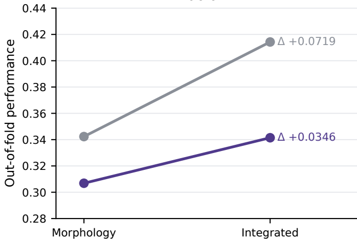
Macro-F1
