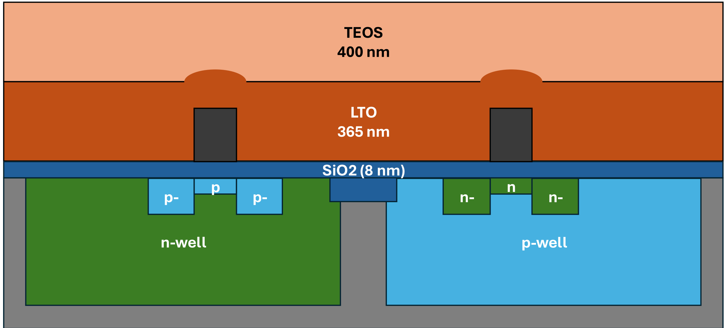
48. LTO + TEOS Deposition
