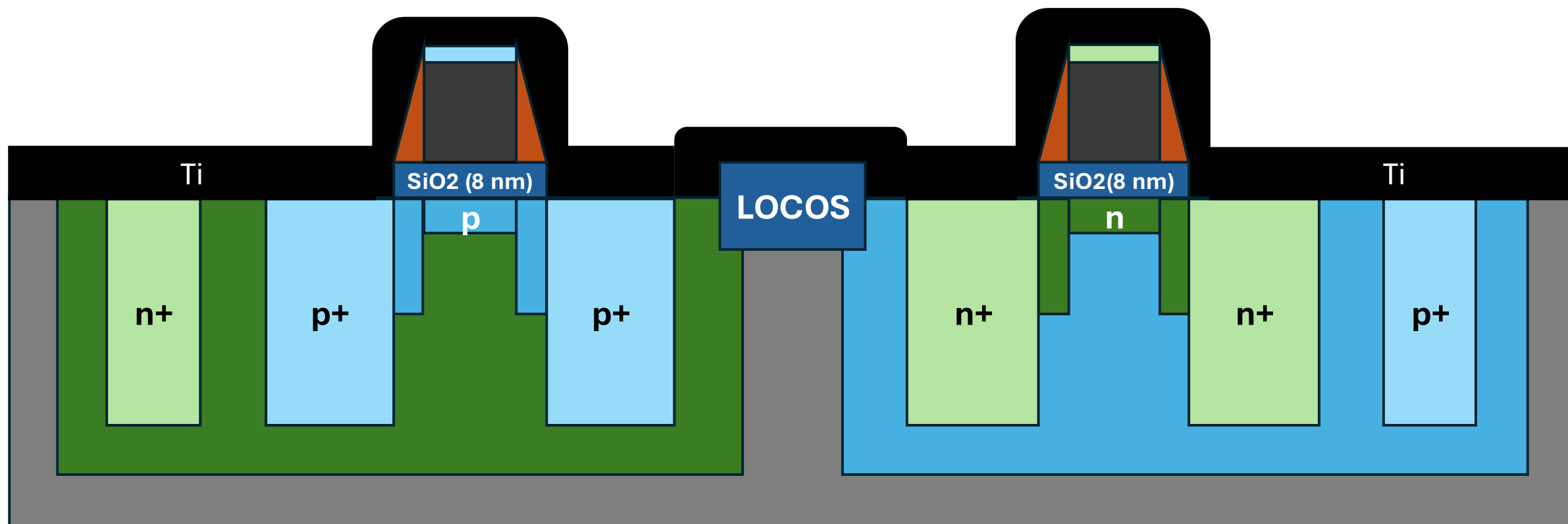
59. Ti Deposition
