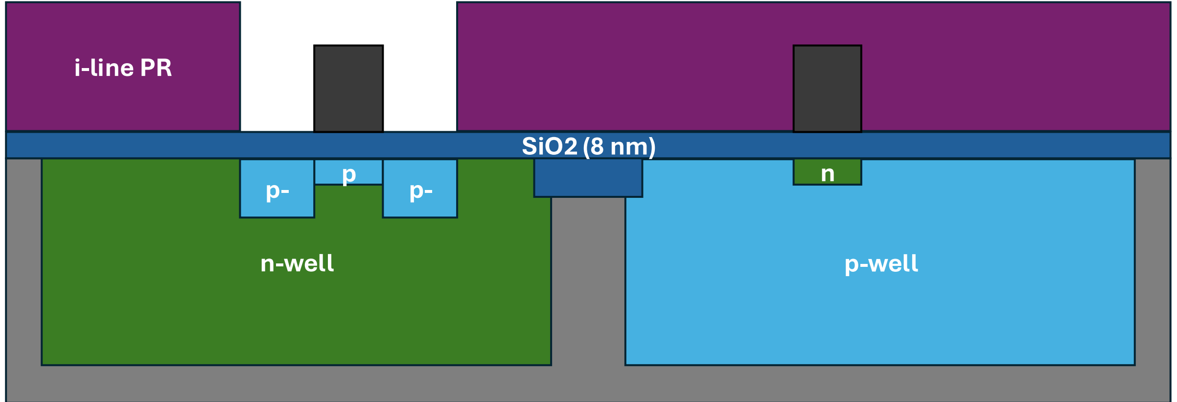
43. PMOS LDD Implant
