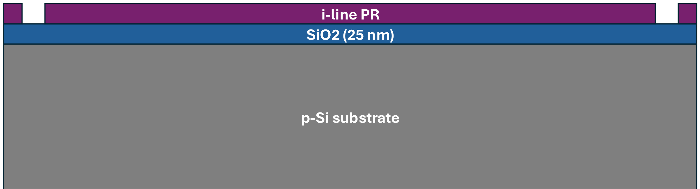
3. Zero Layer Litho
