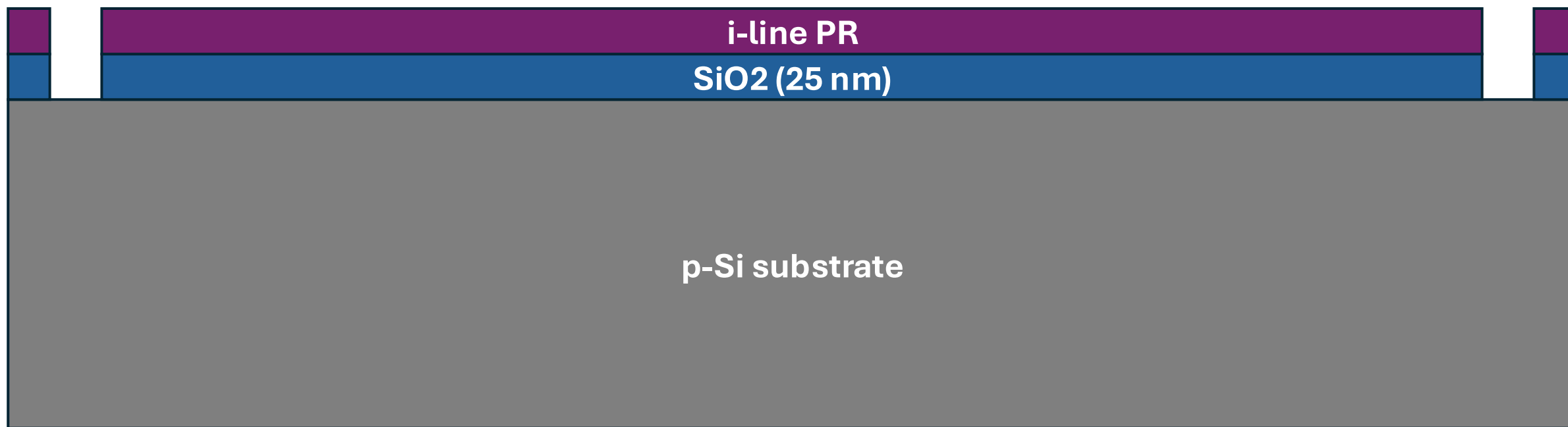
4. SiO2 dry etch
