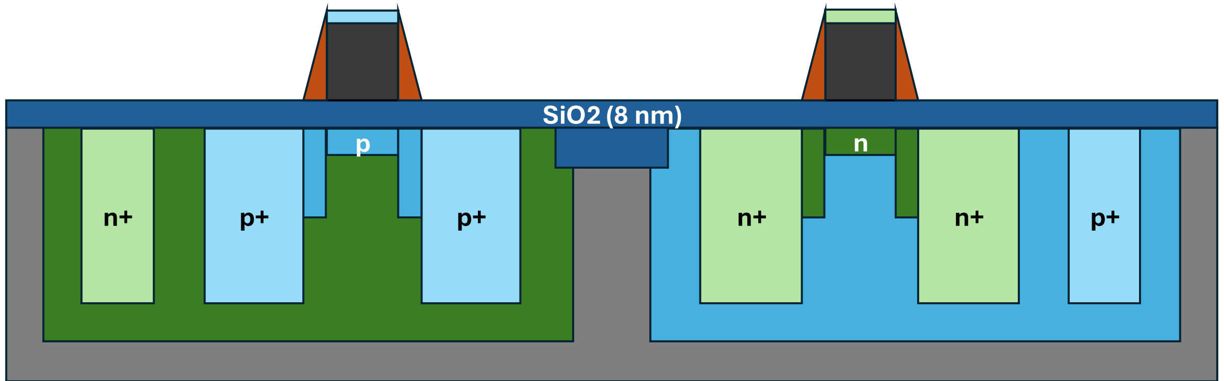
57. PR Strip + S/D Anneal
