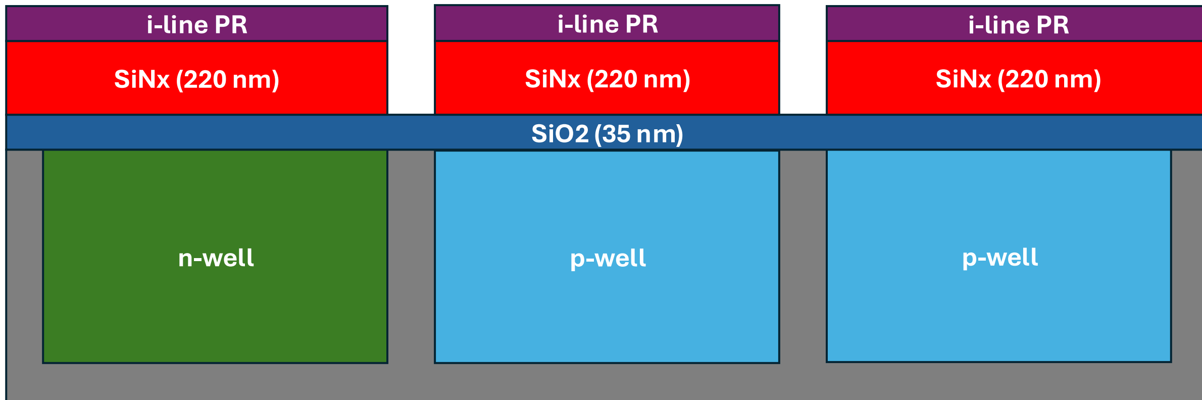
22. Nitride Etch
