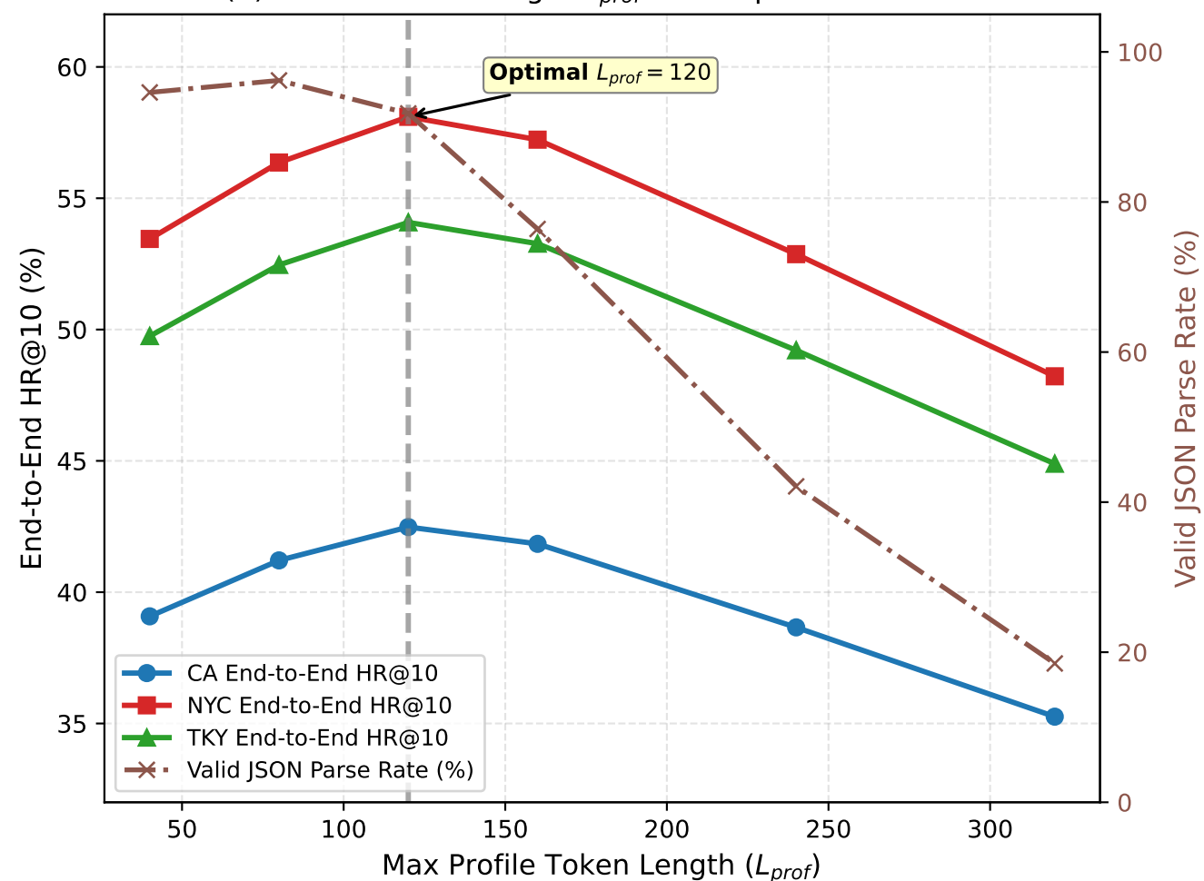
(d) Profile Token Length L_{prof} vs. Output Robustness
