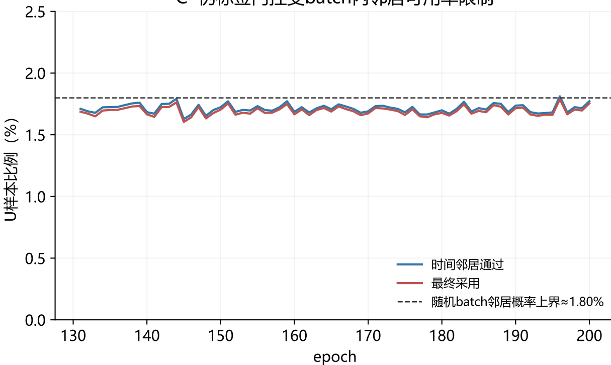
C 伪标签门控受batch内邻居可用率限制
