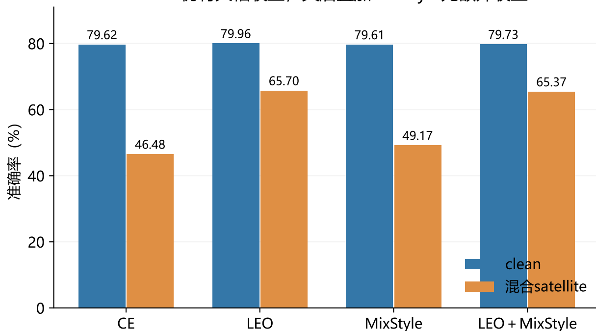
A LEO仍有大幅收益；其后叠加MixStyle无额外收益
