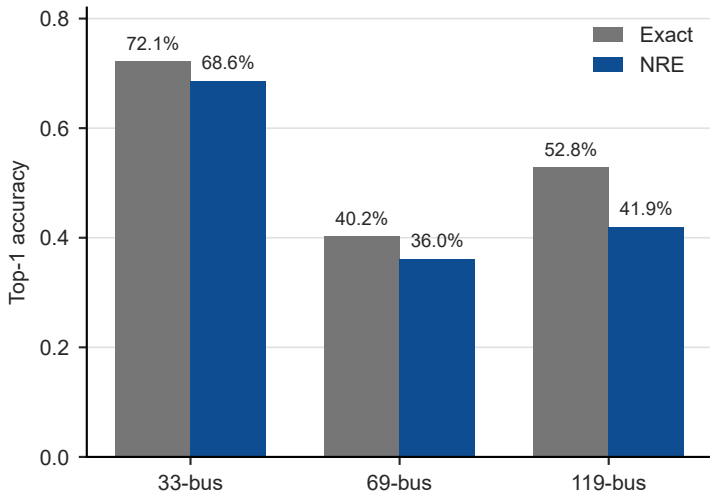
Posterior inference accuracy
