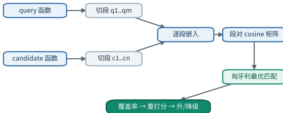
图 3-11 分段验证：切段 → 逐段嵌入 → 匈牙利最优匹配 → 覆盖率
