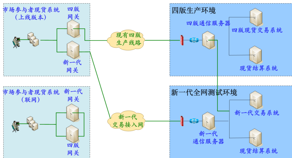
图 3 新一代交易系统全网测试环境示意图
