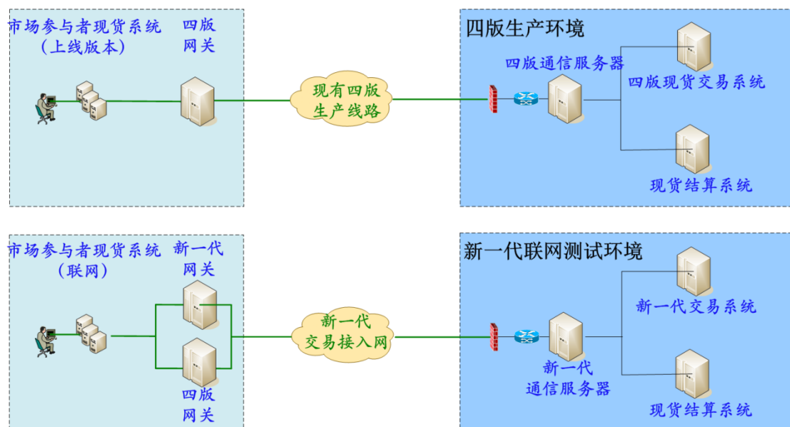
图 2 新一代交易系统联网测试环境示意图
