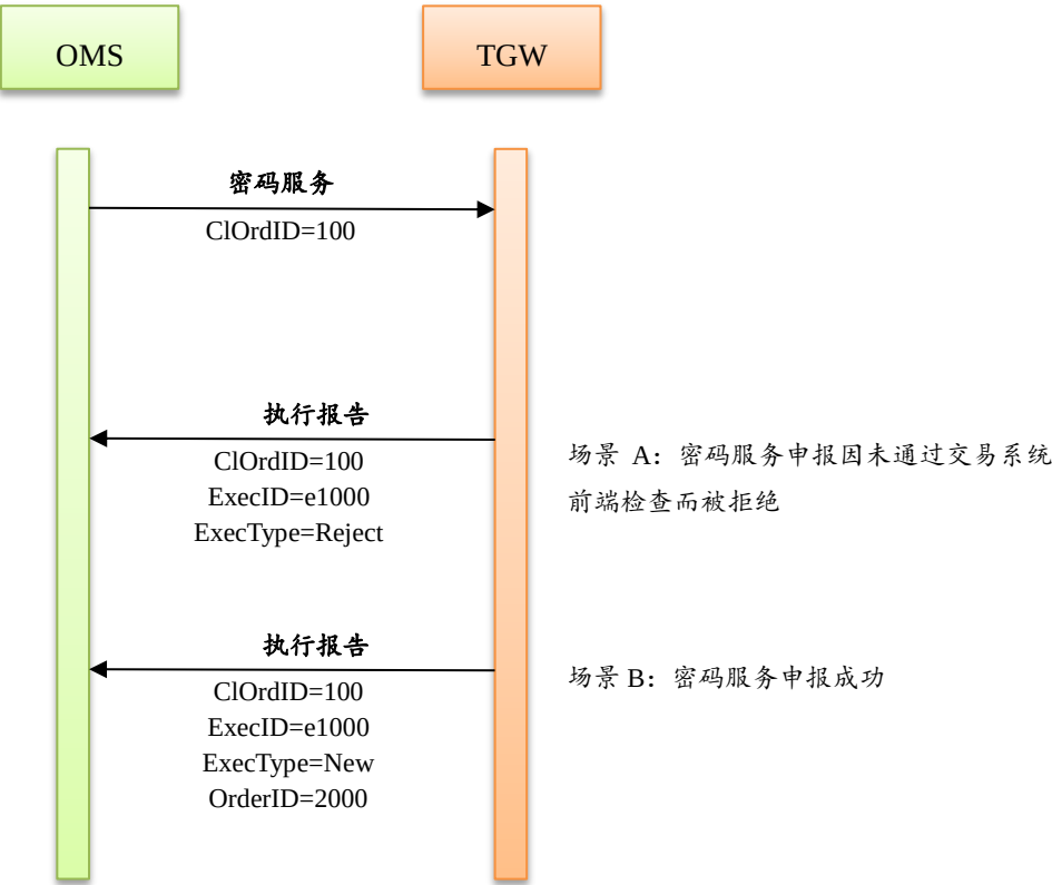
图 3-22 密码服务处理消息流示意图
