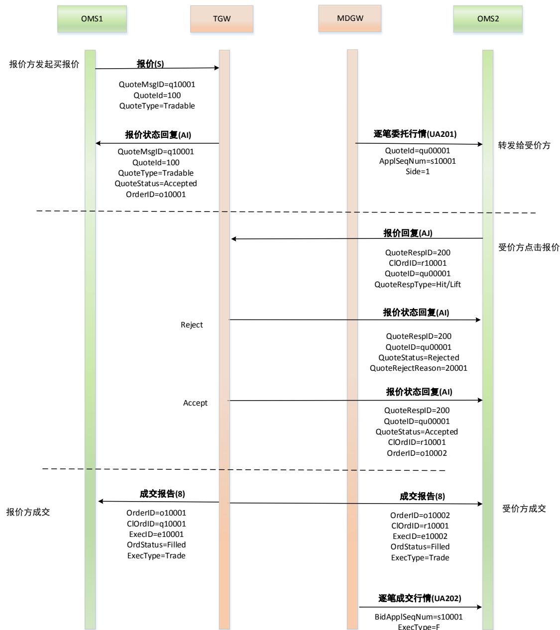
图 3-8 受价方点击成交处理消息流示意图
