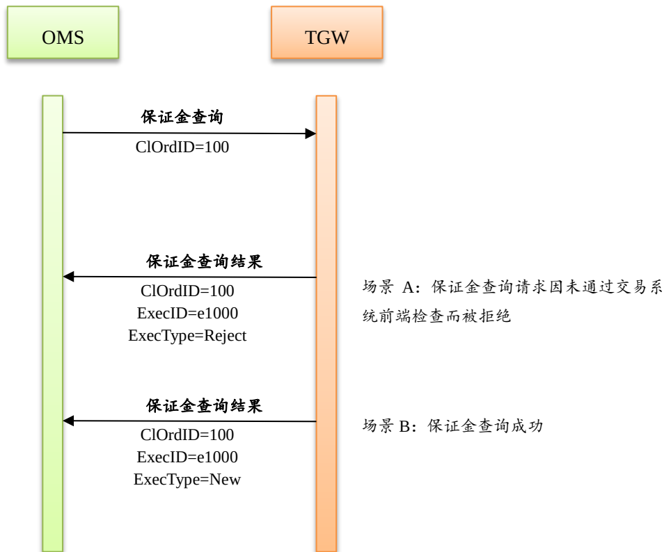
图 3-23 保证金查询处理消息流示意图
