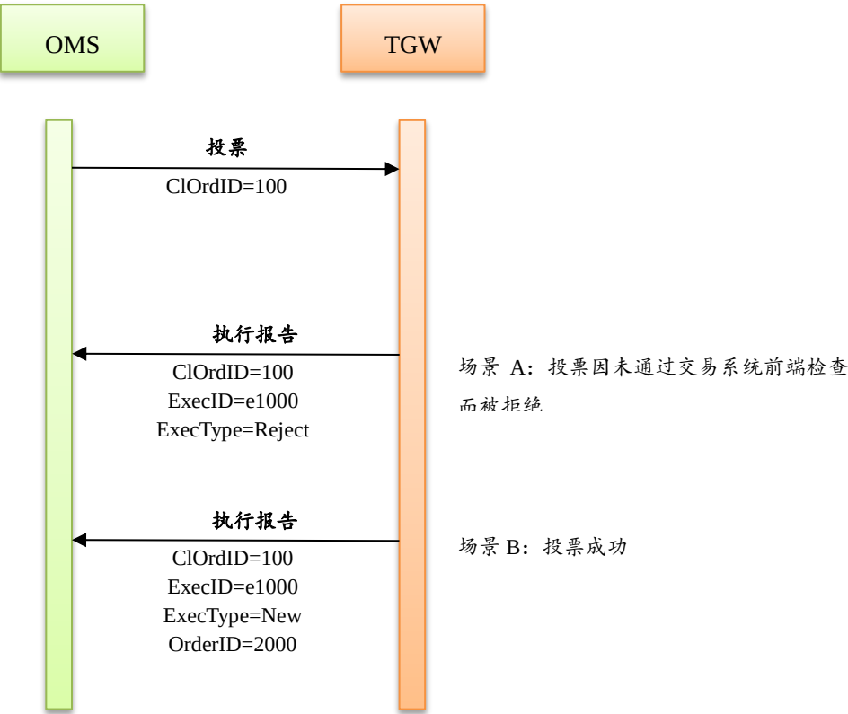
图 3-21 网络投票处理消息流示意图
