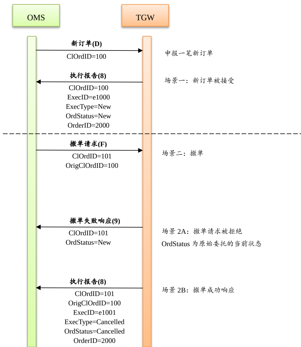
图 3-2 撤单请求消息流示意图
