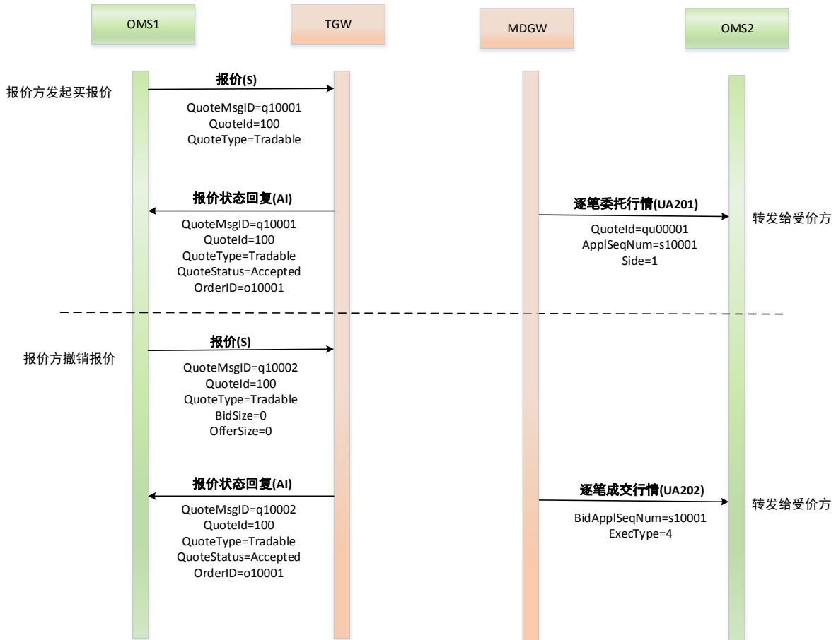
图 3-9 报价方撤销报价处理消息流示意图
