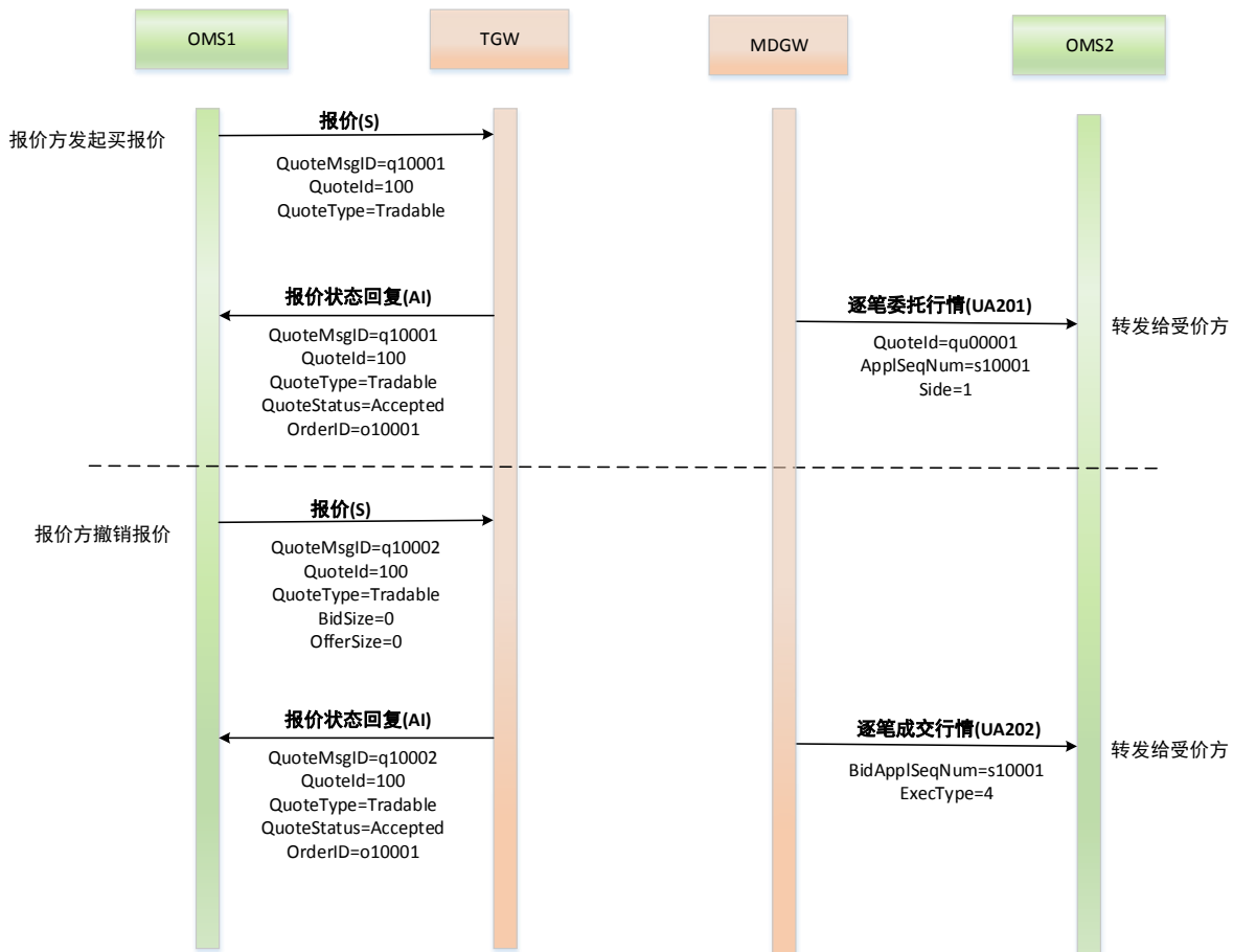
图 3-9 报价方撤销报价处理消息流示意图
