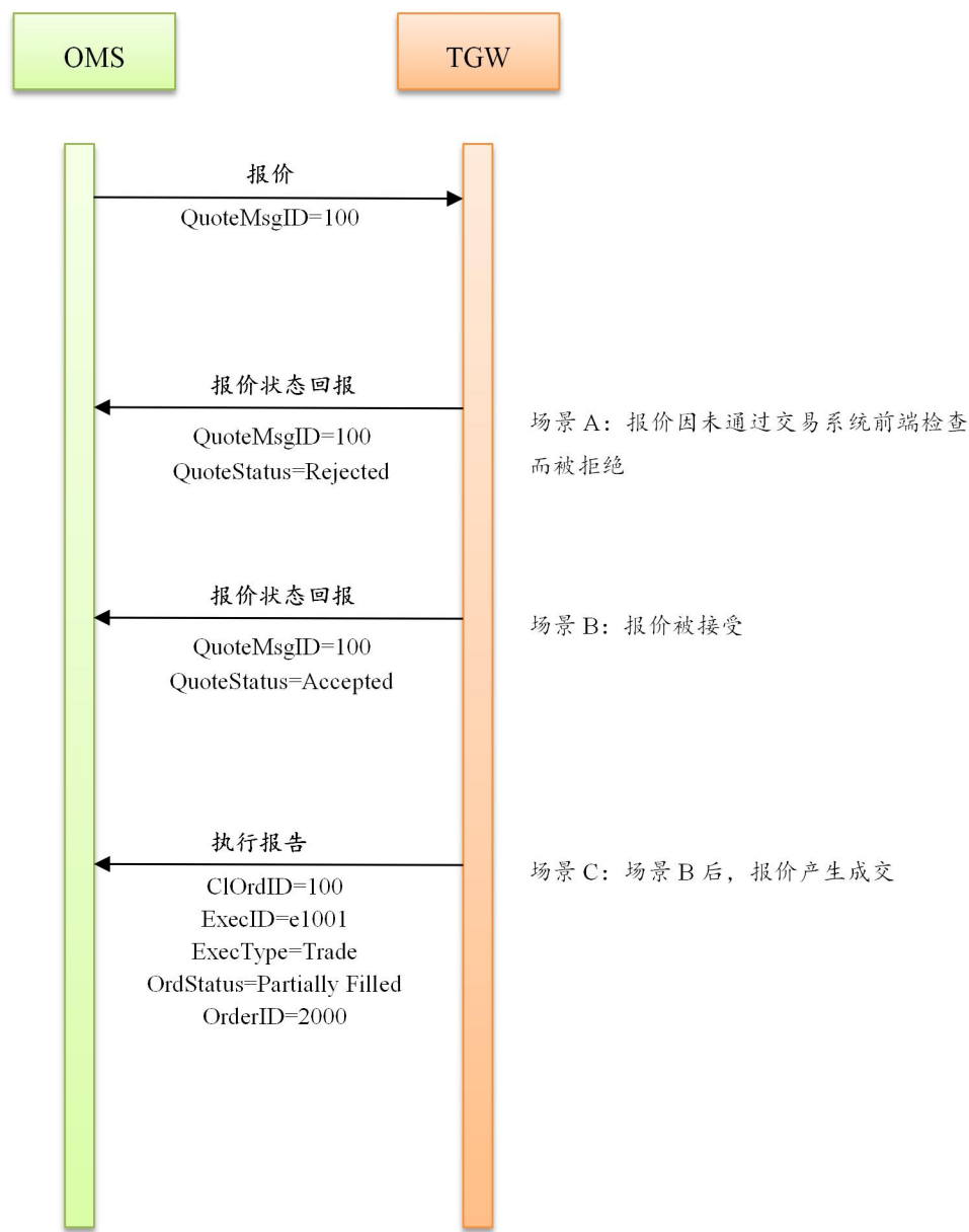
图 3-3 新报价处理消息流示意图
