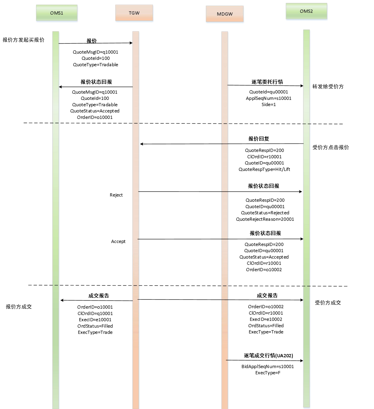
图 3-8 受价方点击成交处理消息流示意图
