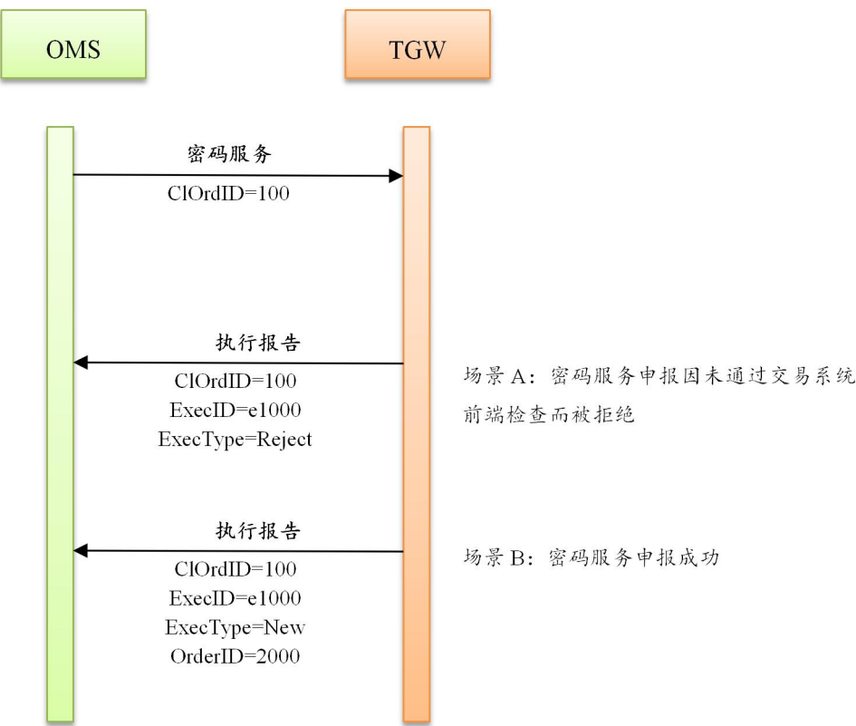
图 3-24 密码服务处理消息流示意图
