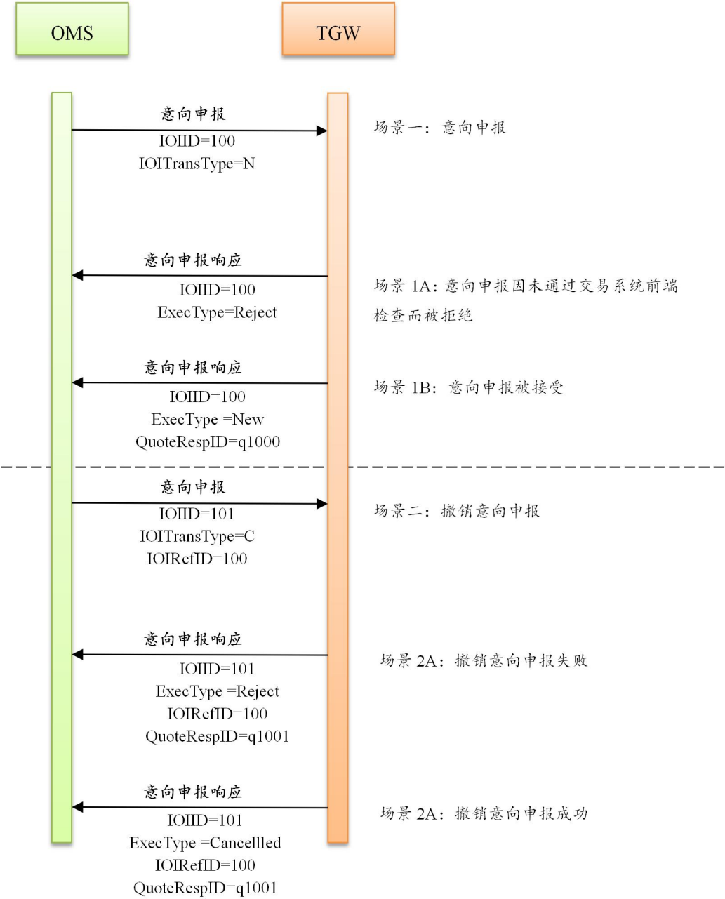
图 3-13 意向申报处理消息流示意图
