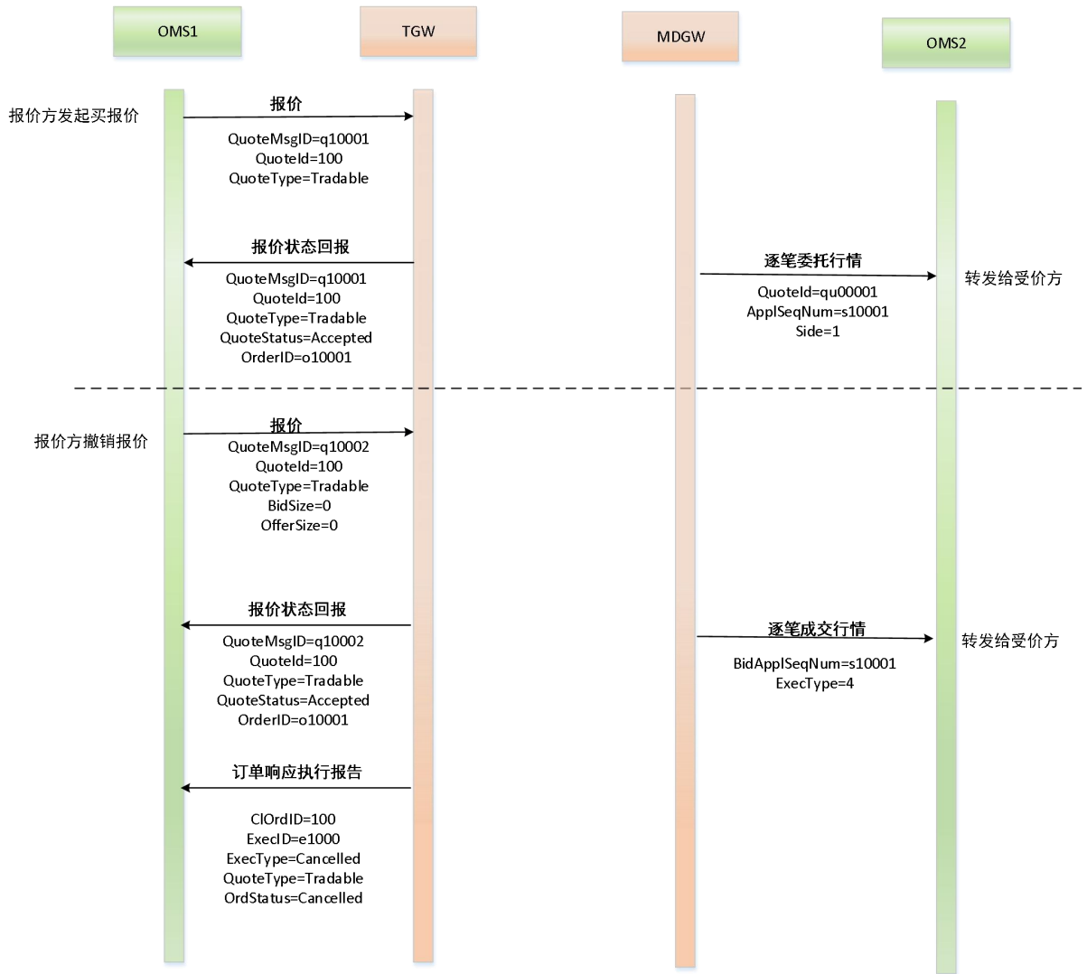
图 3-9 报价方撤销报价处理消息流示意图
