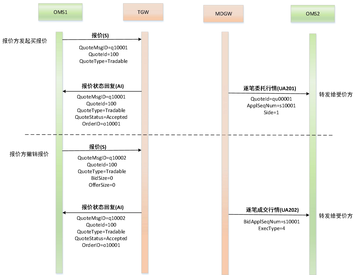
图 3-9 报价方撤销报价处理消息流示意图
