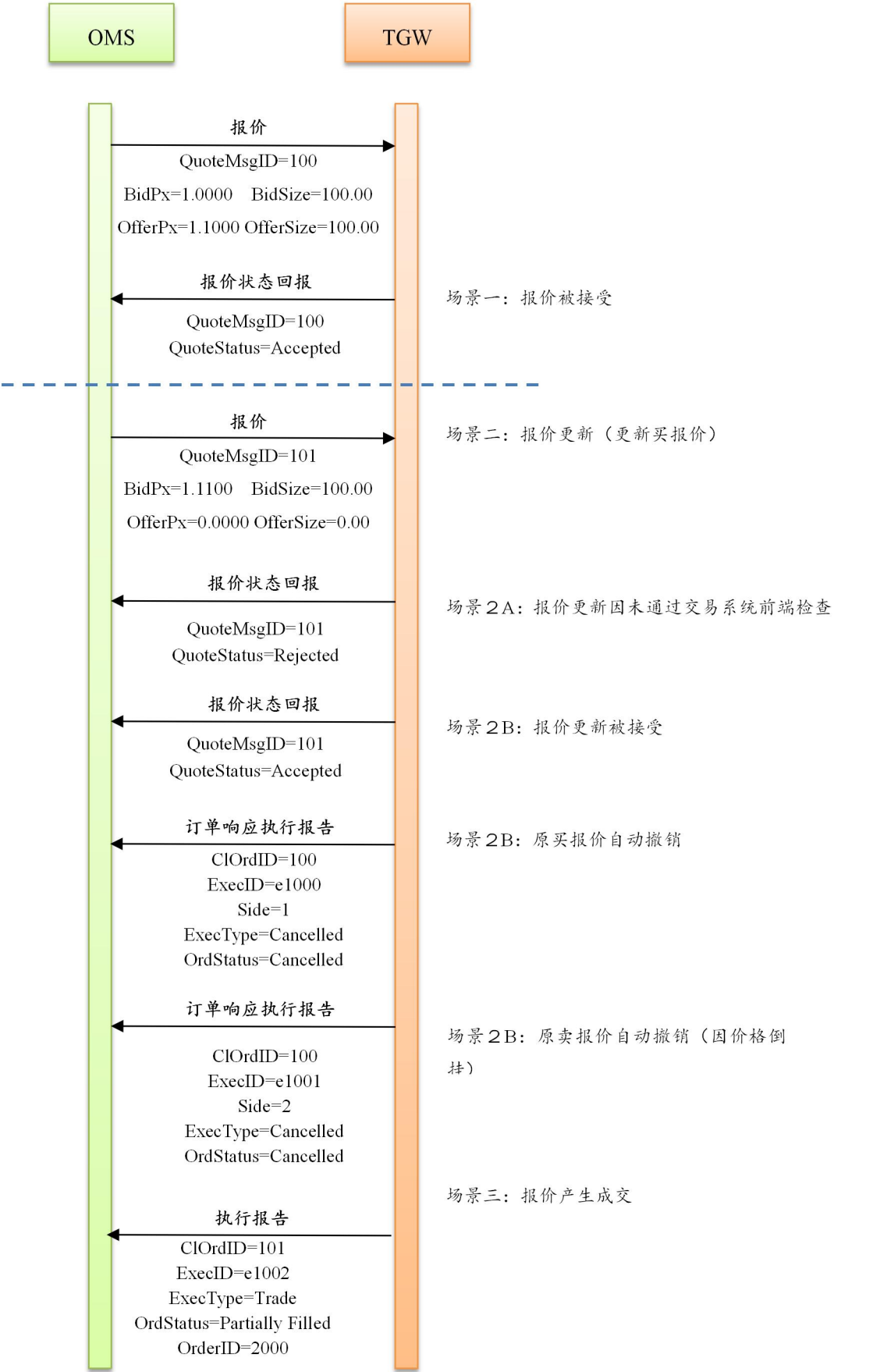
图 3-6 更新单边报价（情形三）处理消息流示意图
