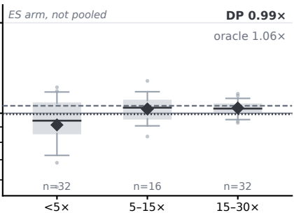
DeiT-S
