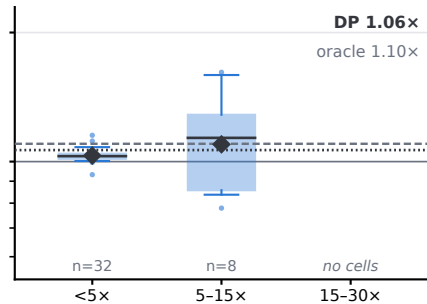
VGG-16
