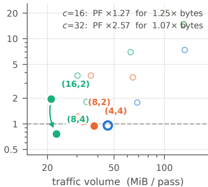
VGG-16
