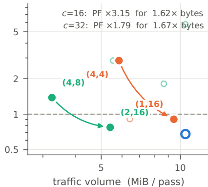
DeiT-S
