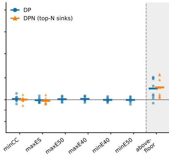
VGG-16 (16,4,4)
