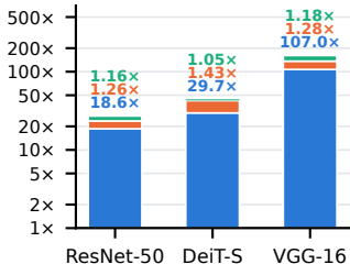
p99 delay
