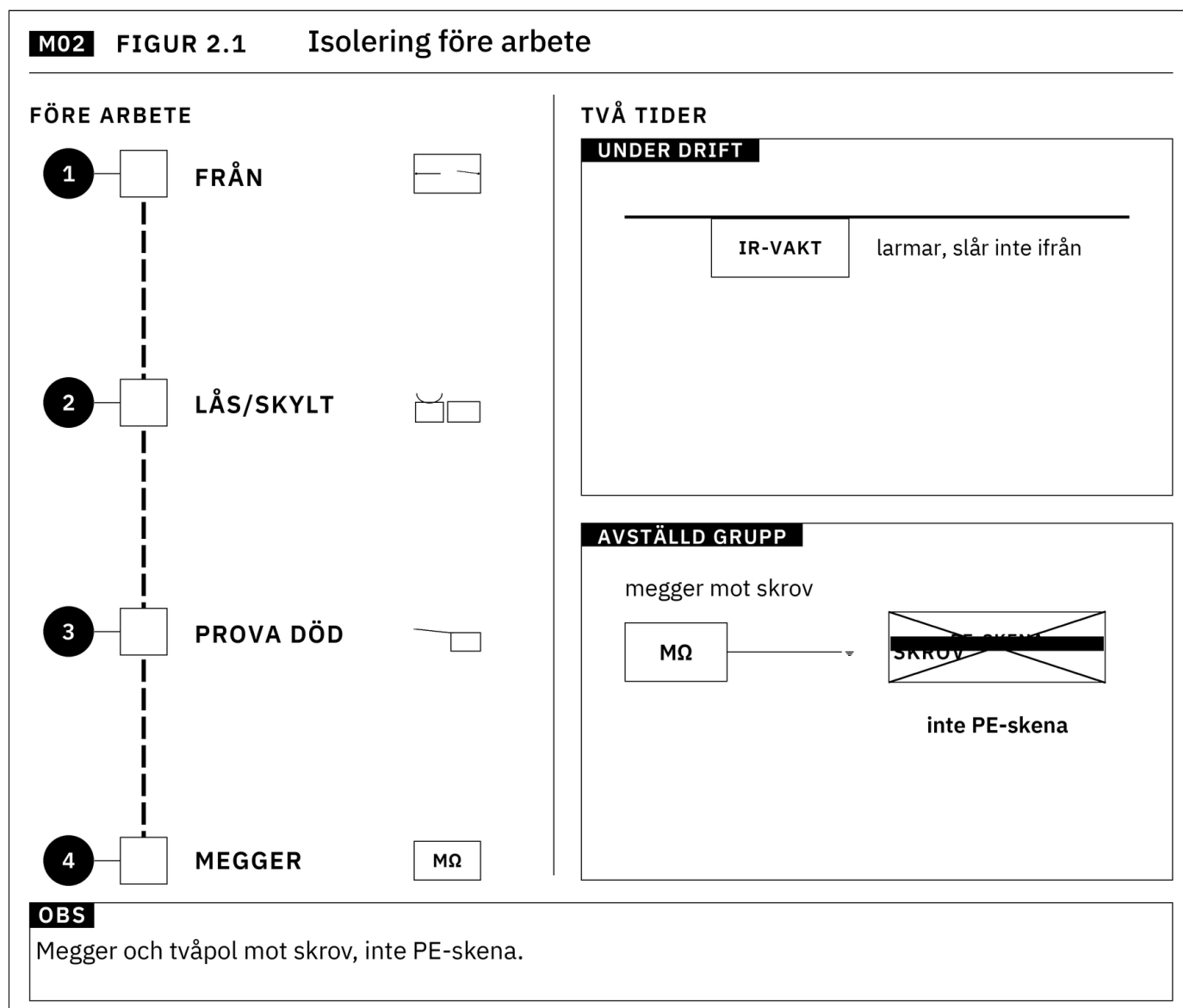
Figur 2.1 Isolering före arbete (bok). Kedja från–lås–prova–megger. 1 MΩ = upplysning.
