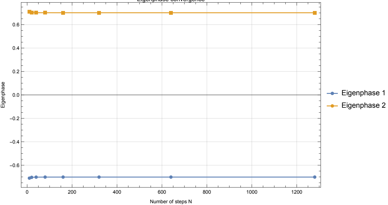
Eigenphase convergence
