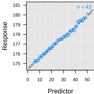
-- L pc Rank 1: y = 174.51 + 0.1073 \cdot x
