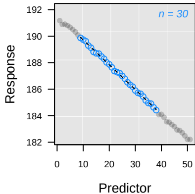
-- L_{pc} Rank 1: y = 191.60 - 0.1877 \cdot x
