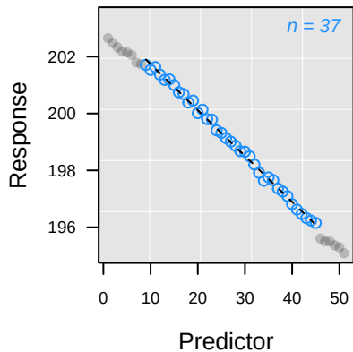
-- L_{pc} Rank 1: y = 203.35 - 0.1614 \cdot x
