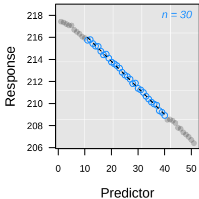
-- L_{pc} Rank 1: y = 218.63 - 0.2406 \cdot x
