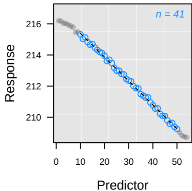
-- L pc Rank 1: y = 216.93 - 0.1534 \cdot x
