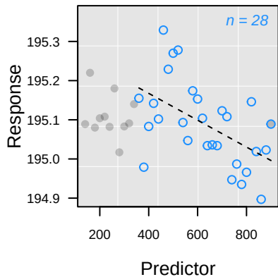
-- L_{pc} Rank 1: y = 195.30 - 0.0003 \cdot x
