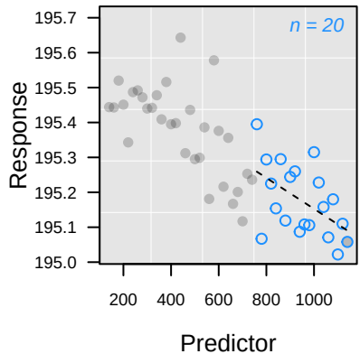
-- L_{pc} Rank 1: y = 195.60 - 0.0004 \cdot x
