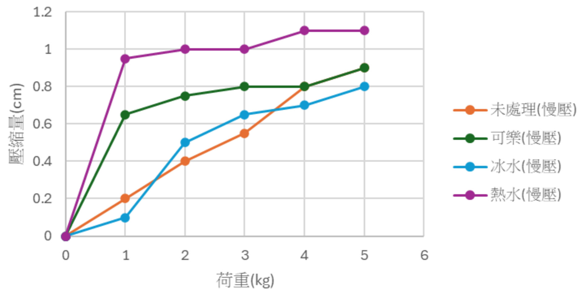
壓縮量與荷重之關係
