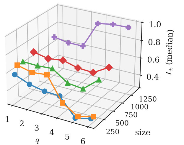
Cheng2020-Anchor
