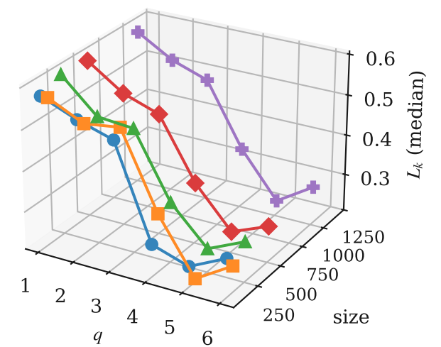
Cheng2020-Attn
