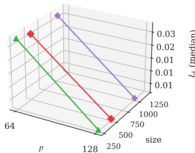
TCM
