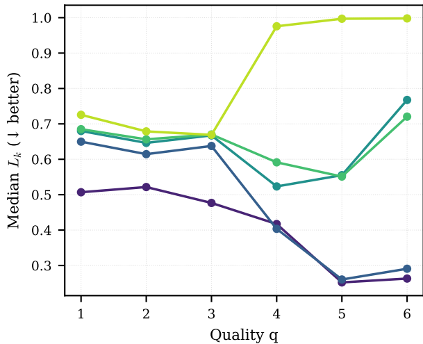
Cheng2020-Anchor
