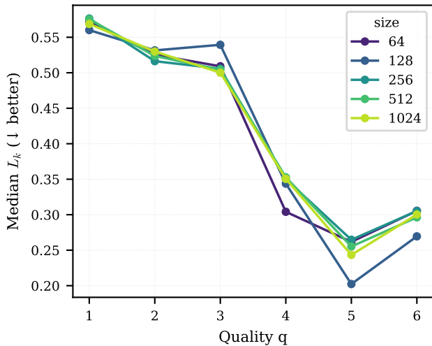
Cheng2020-Attention
