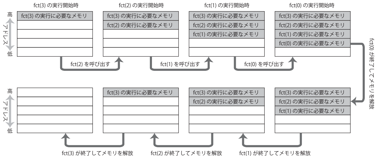
図 5: 関数 fct(3) が呼び出され、終了するまでのメモリの割り当てと解放
