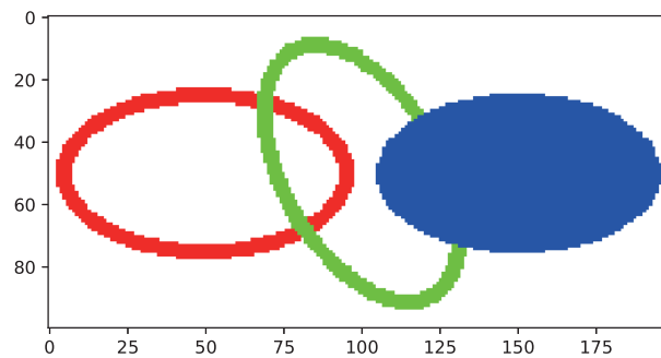
図 15: 楕円の描画
