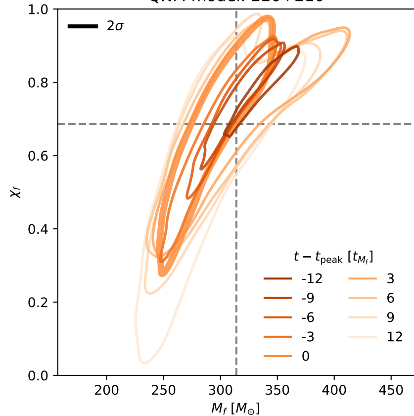
QNM model: 220+210
