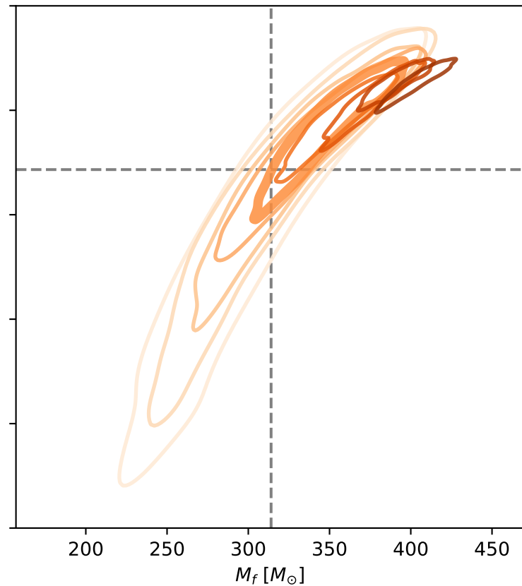
QNM model: 220+221
