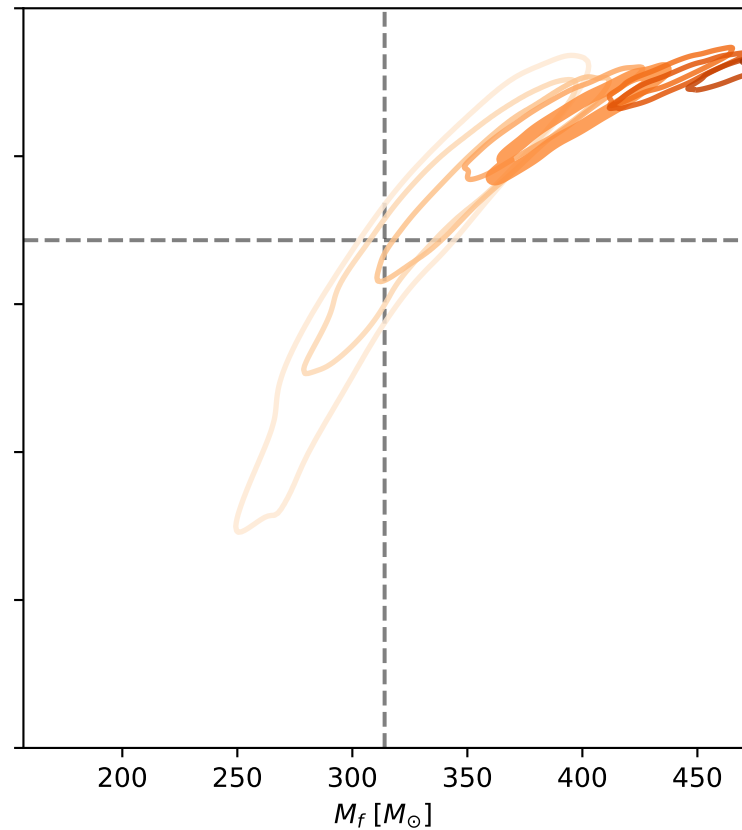
QNM model: 220
